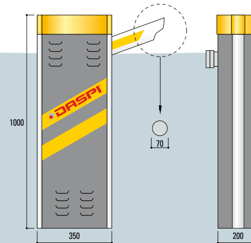
LUNGHEZZA MASSIMA ASTA DELLA BARRIERA ELTRA
